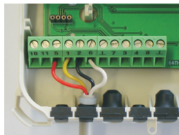
Двухпроводное подключение термометров
